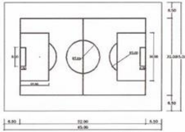
แปลนสนามฟุตบอล 7 คน แบบไม่ปูหญ้า ขนาดสนาม 1 : 500
