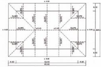
แปลนพื้นที่แสดงความลาดเอียง ขนาดสนาม 1 : 500
