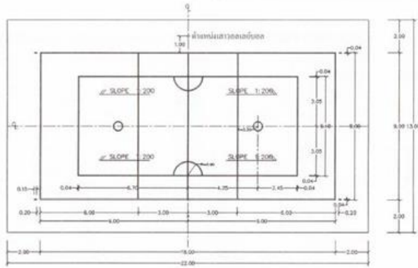
แปลนสนาม ขนาดสนาม 1 : 100
